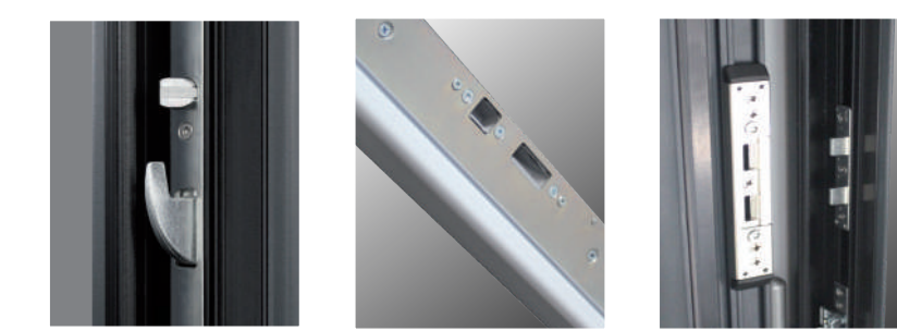
Serrure 5 points à crochets | Gâche filante | Pièces anti-dégondage haute et basse
